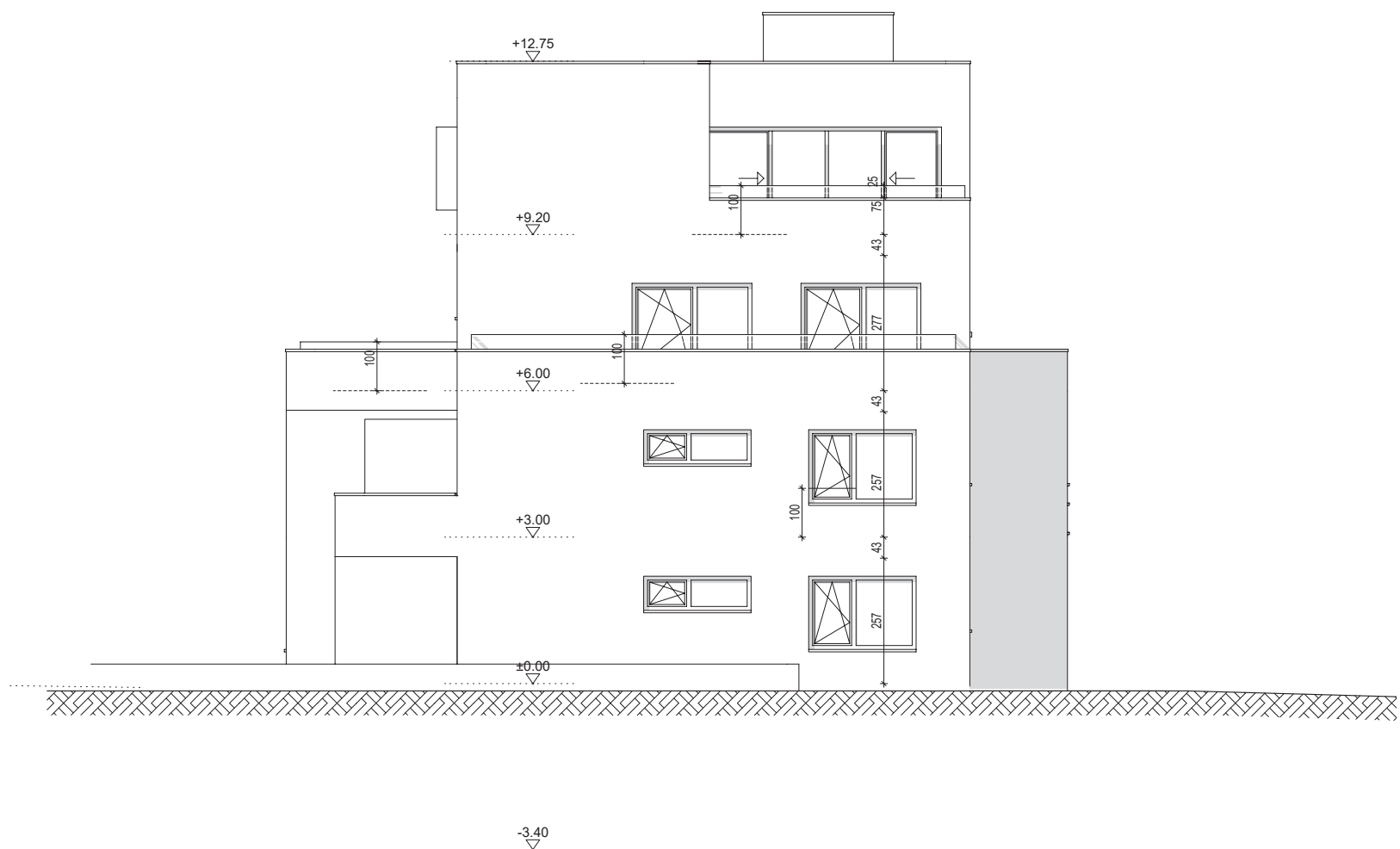
Façade est E 100
