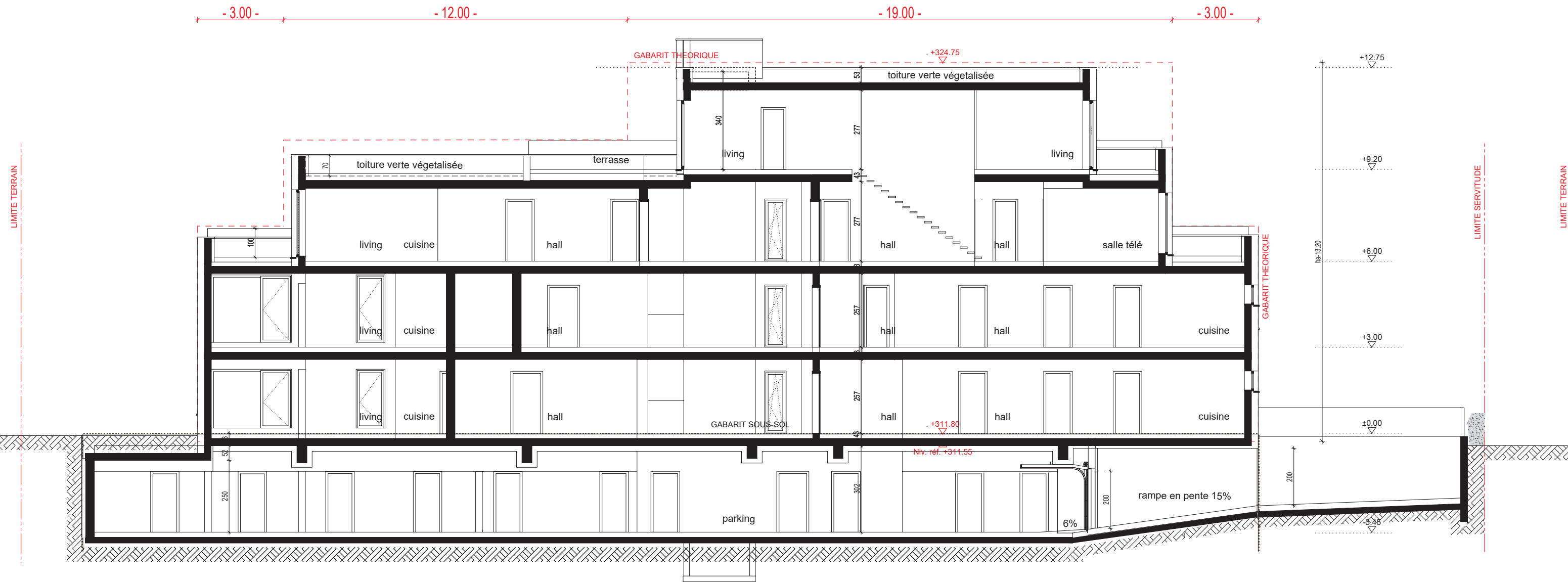
Coupe A-A E 100
